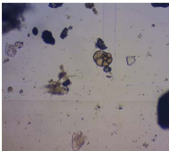
Globigerina sp.
