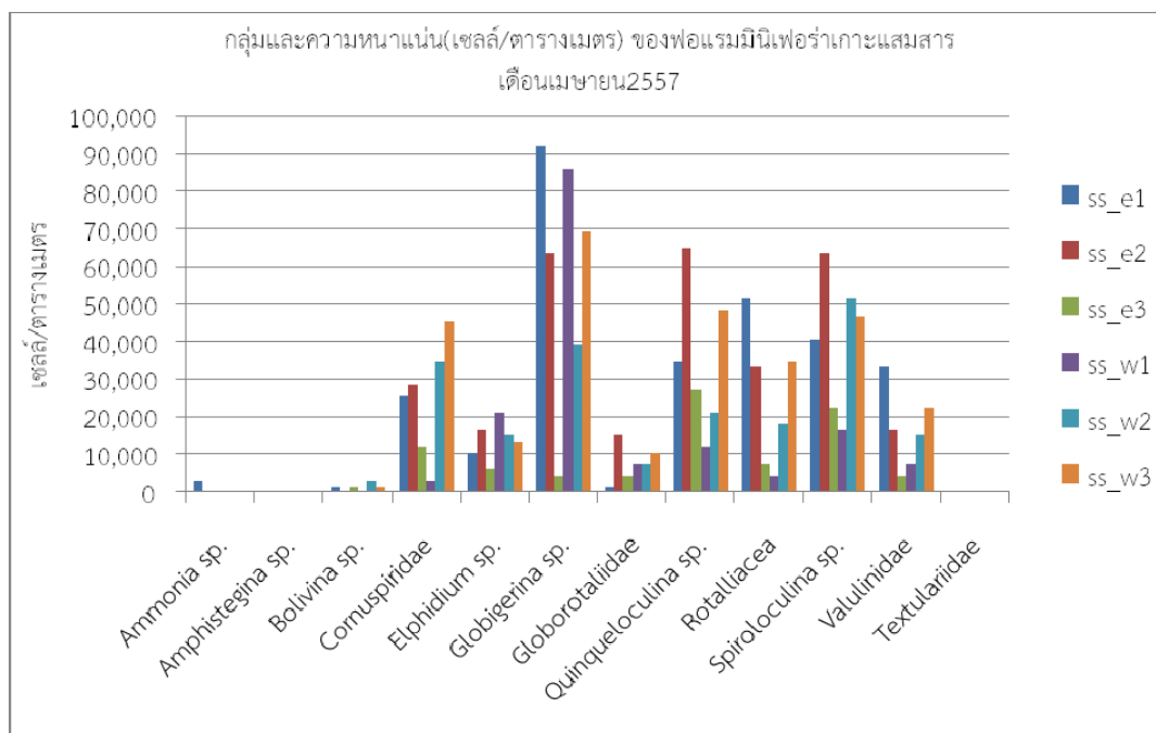
รูปที่ 7 กลุ่มและความหนาแน่น (เซลล์/ตารางเมตร) ของกลุ่มฟอแรมมินิเฟอรา เกาะเสมสาร เดือนเมษายน 2557
