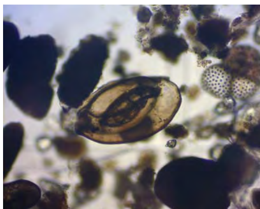
Spiroloculina sp.
